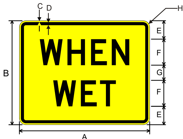
W8-5P
