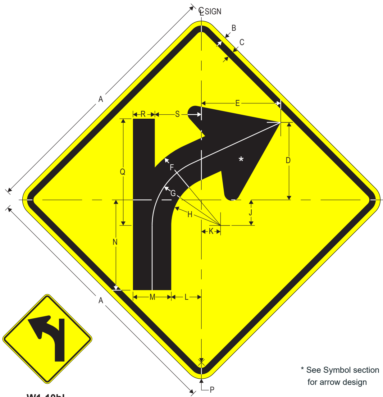
W1-10bL
