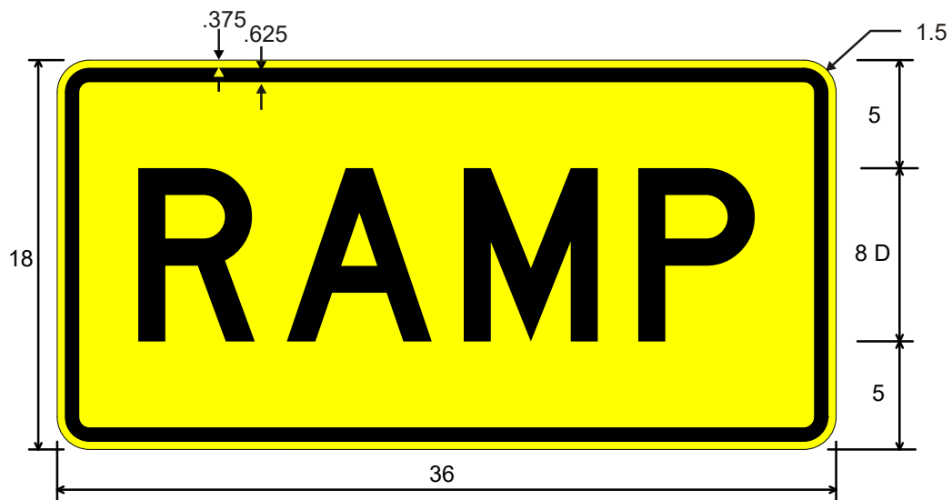
W13-4aTP RAMP
