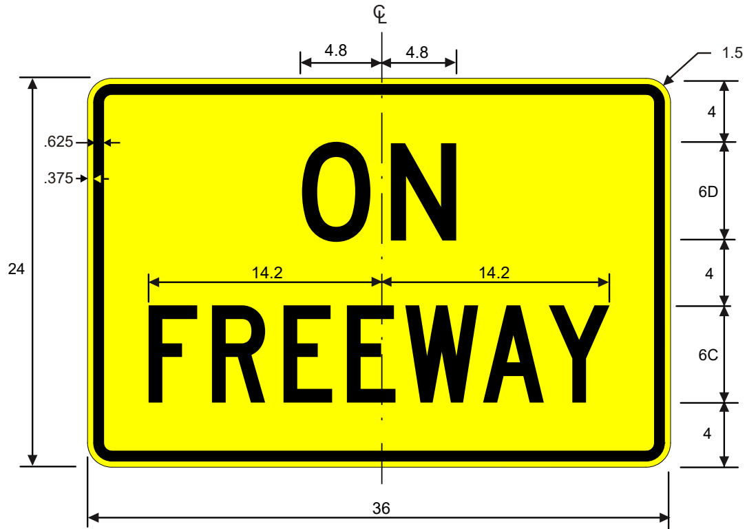
W13-4bTP
