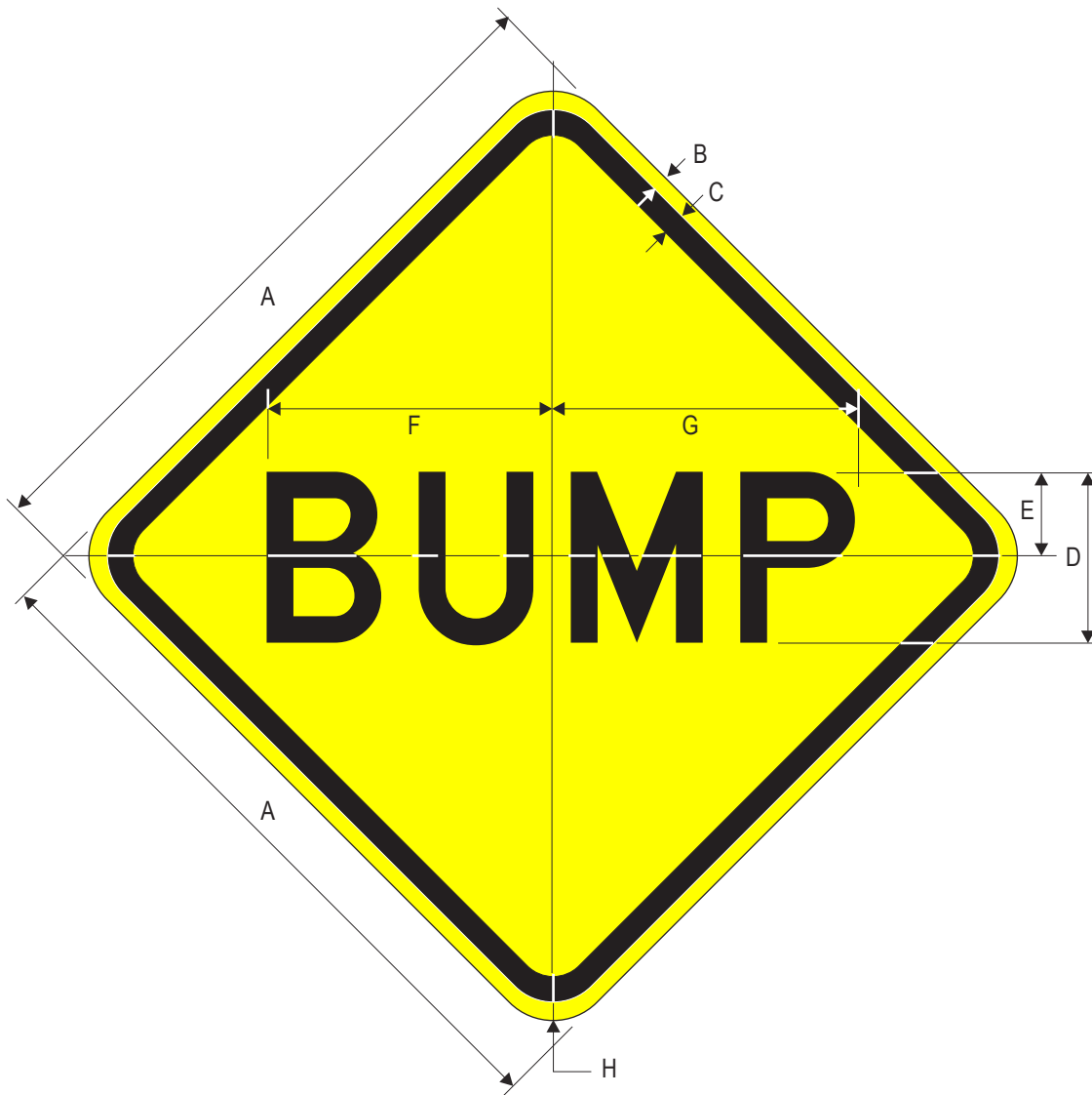
W8-1 BUMP
