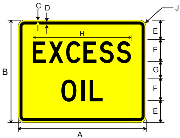
W8-5cP
