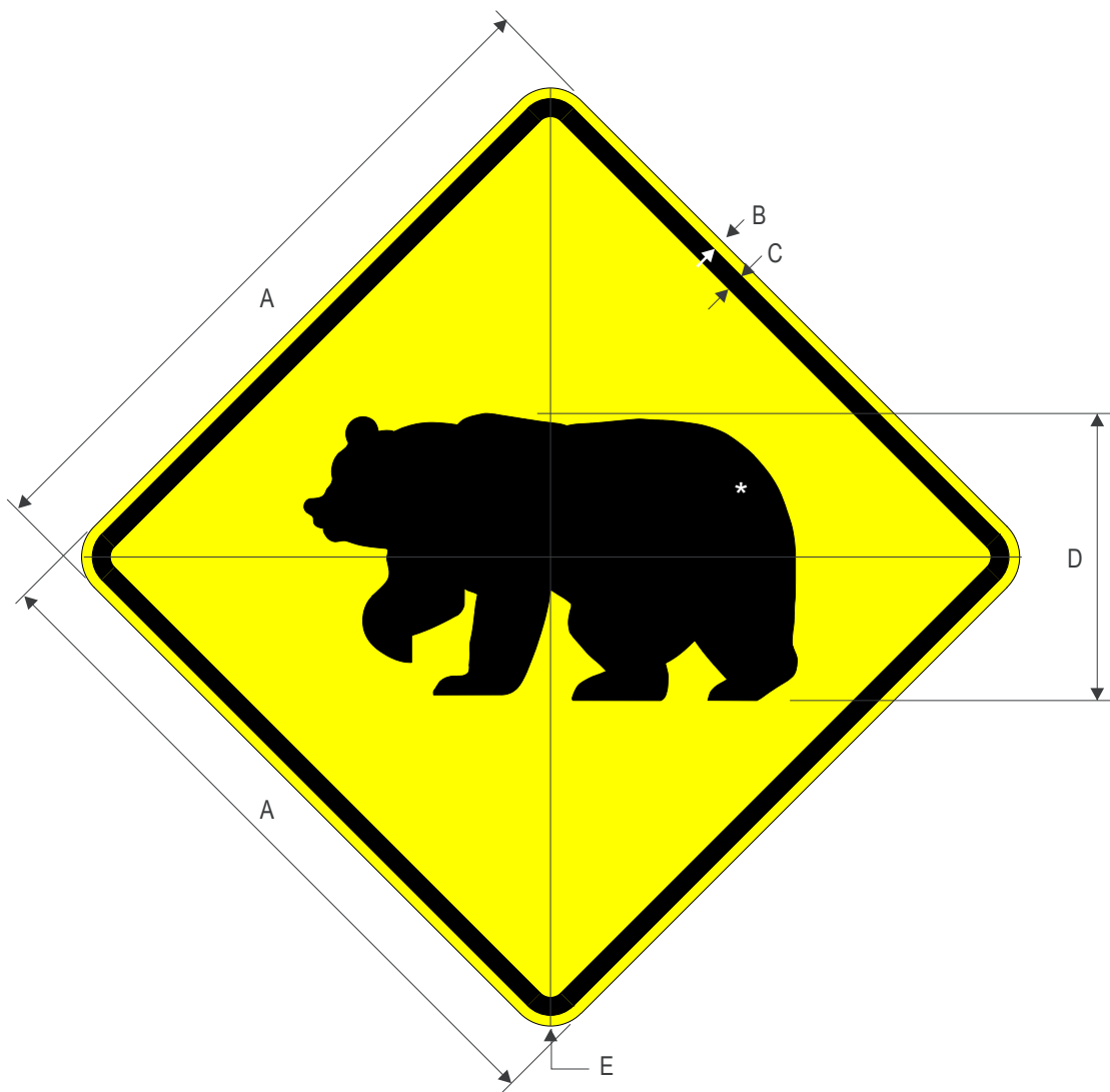
W11-16 (Bear)
