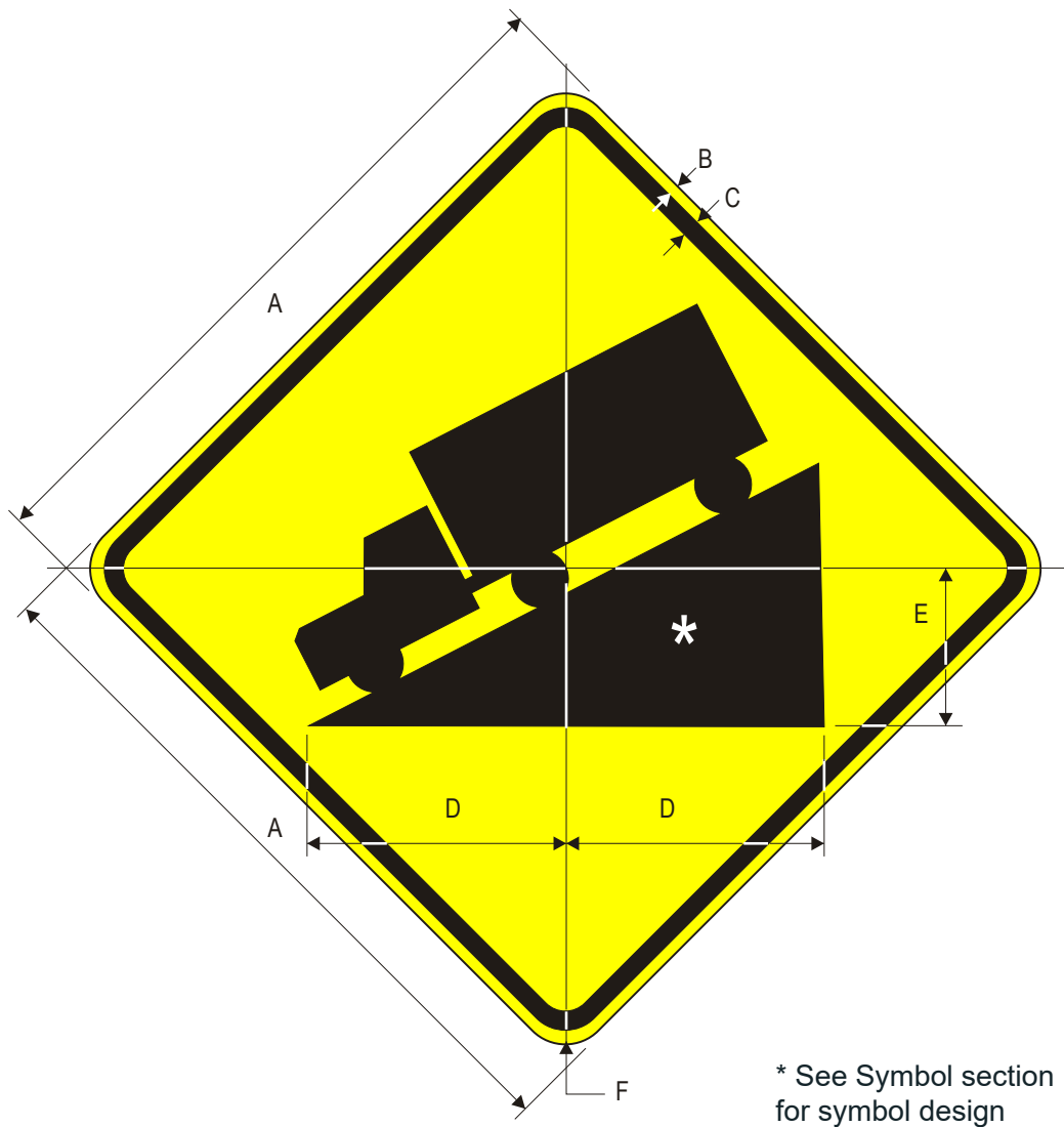
W7-1 Hill (Symbol)
