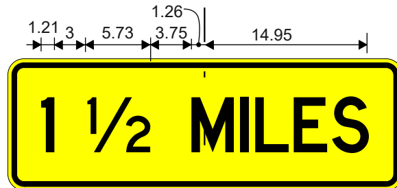
W16-3aTP (3)
