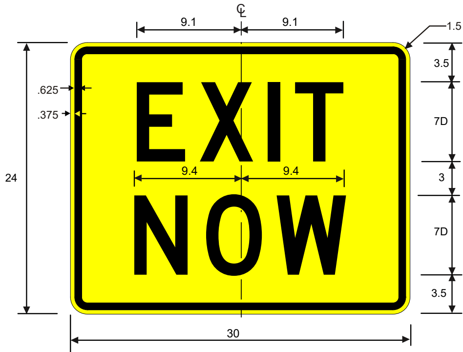
W13-4cTP
