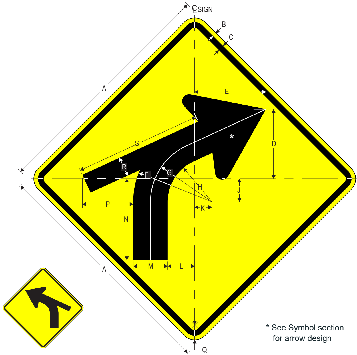
W1-10cL
