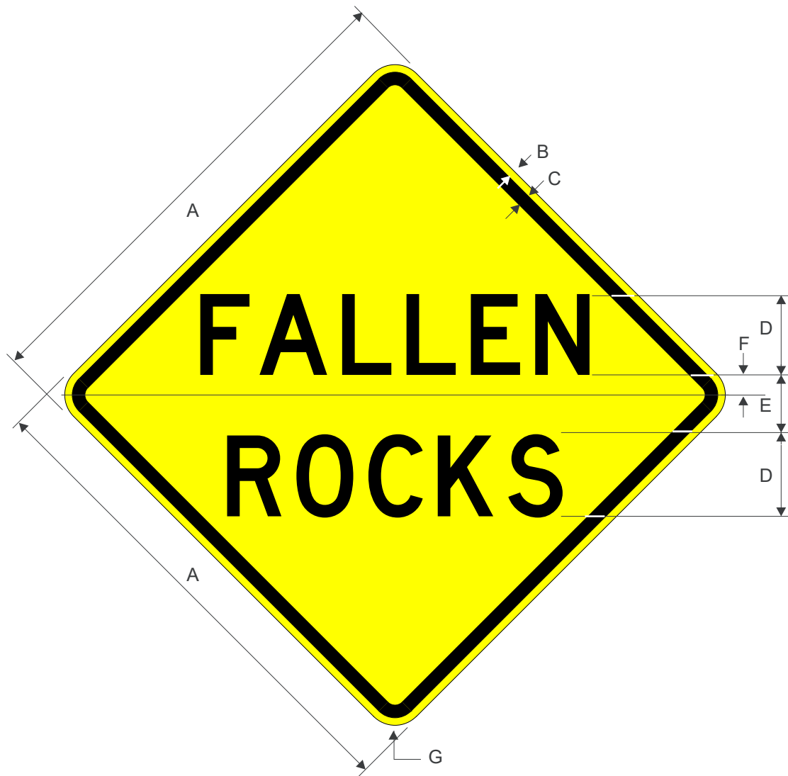
W8-14 FALLEN ROCKS
