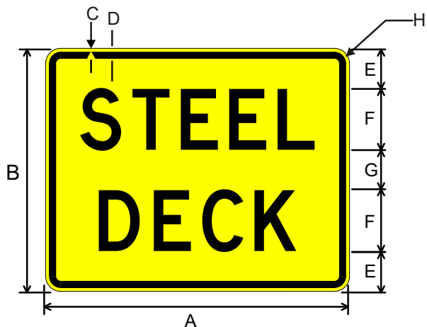
W8-5bP
