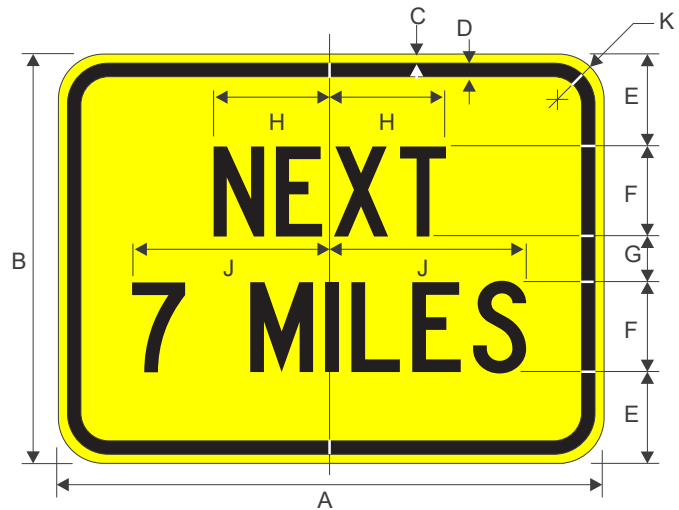
W7-3aP W7-3aP _ NEXT X MILES
