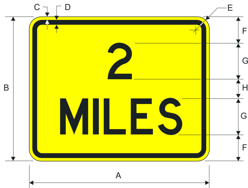
W16-3P (4)
