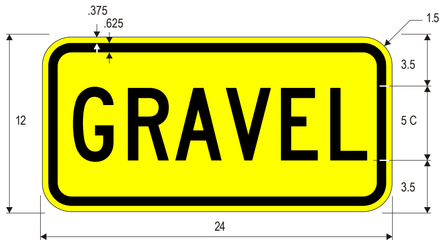
W7-4eP GRAVEL (Plaque)
