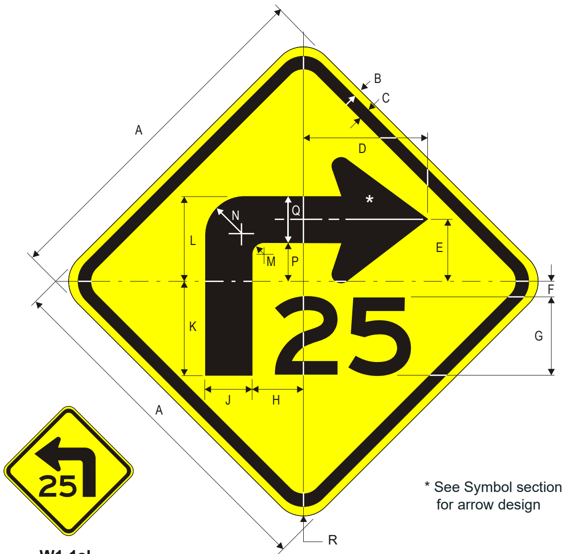
W1-1aL
